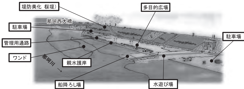
戸多地区かわまちづくり 整備イメージ
