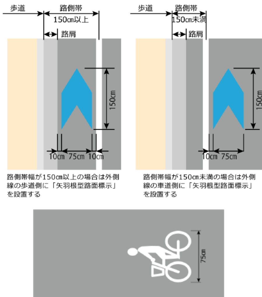
図V-4 矢羽根型路面表示とピクトのデザイン・寸法
