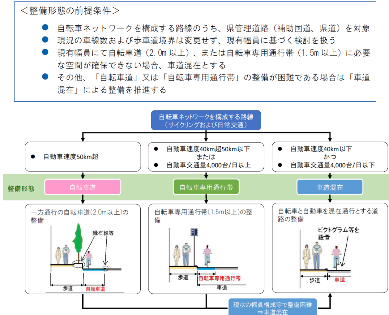
図 V—3 自転車通行空間の整備形態の考え方
