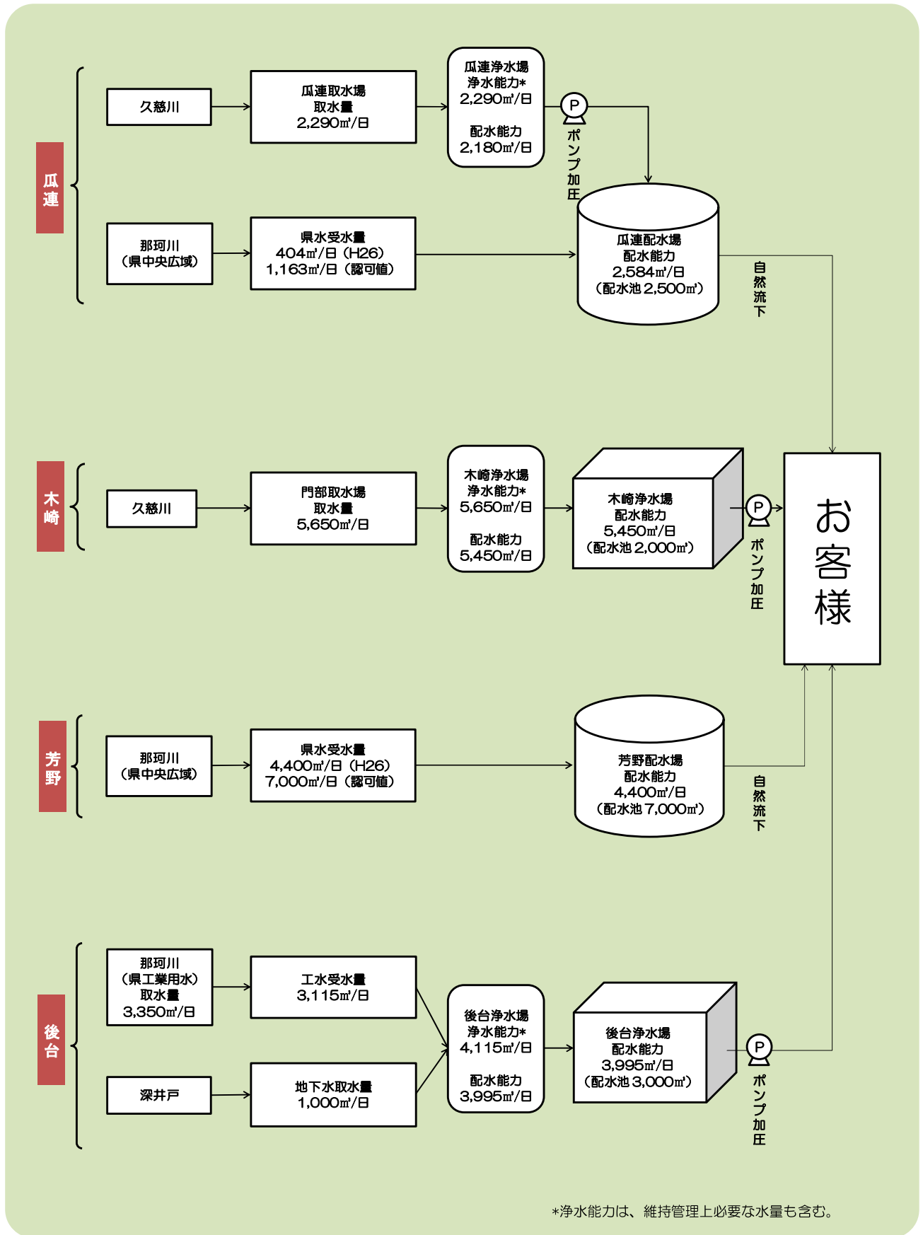
図 3-4 浄水フロー
